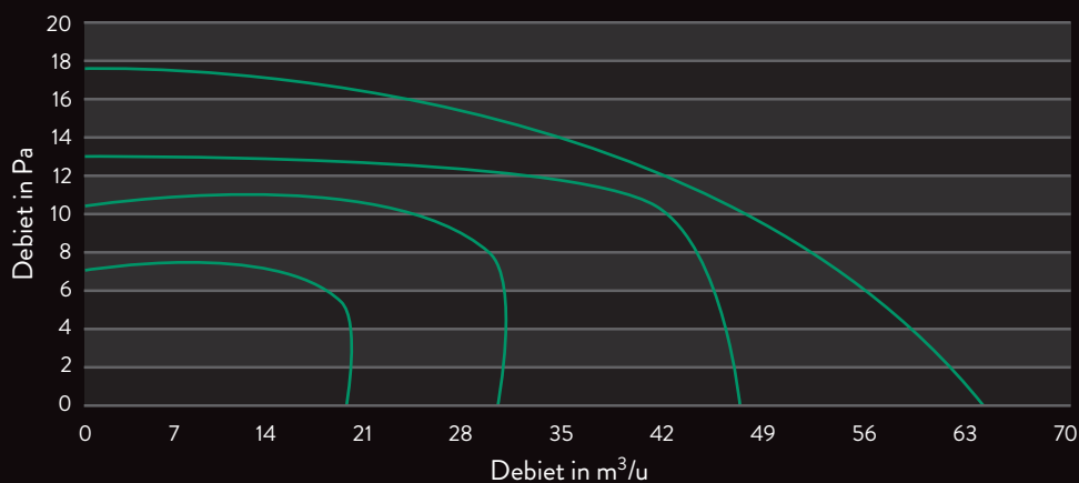
Prestatiecurve ventilators met constant volume: Debiet vs. druk
